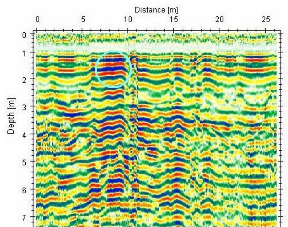
Figura 3. Exemplo de seção GPR obtida na área (círculo indica Tanque).
