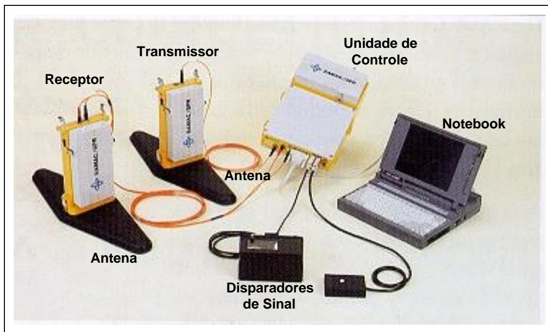
Figura 4. Equipamento Ramac/GPR (Fonte: Malä Geoscience).
