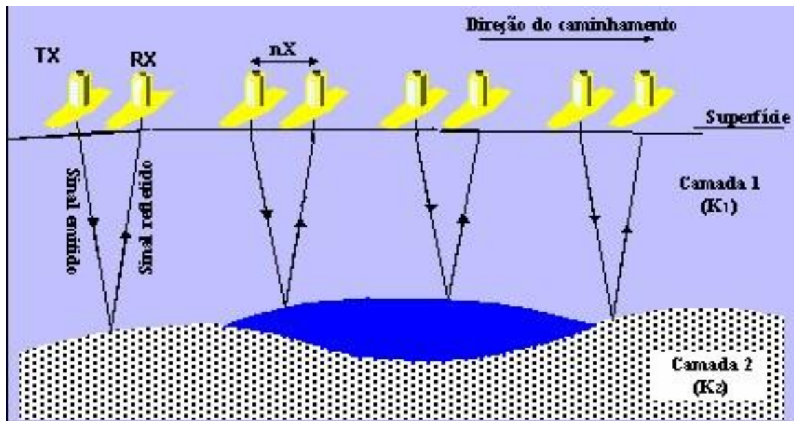
Figura 2. Esquema de emissão e reflexão do sinal GPR em subsuperfície.
